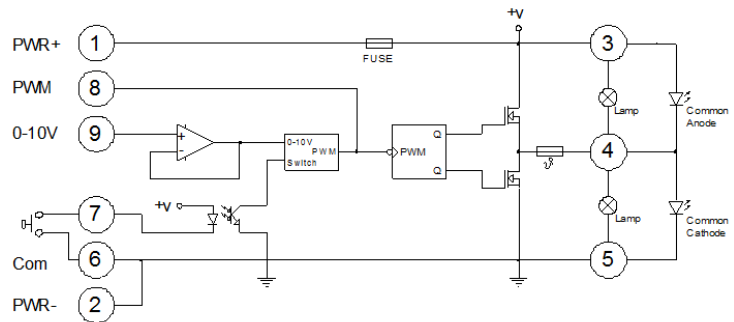
Schema a Blocchi
