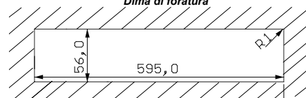
Dima di foratura
