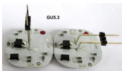
Spot 29 - Attacco centrale e laterale GU5.3
