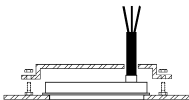
Sistema di fissaggio, posteriore
