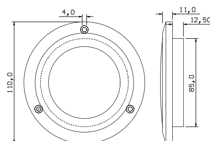
Dimensione lampada con cornice, AV0409
