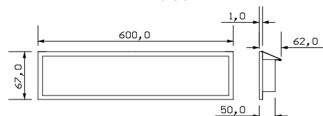
Dima di foratura
