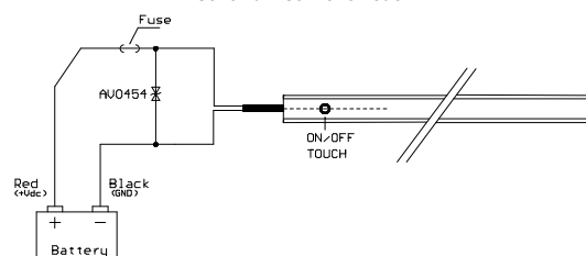
Schema inserzione Touch
